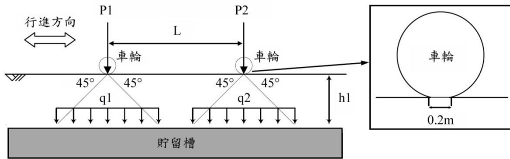
圖-解 3.7.2-3 車輛載重之構想
