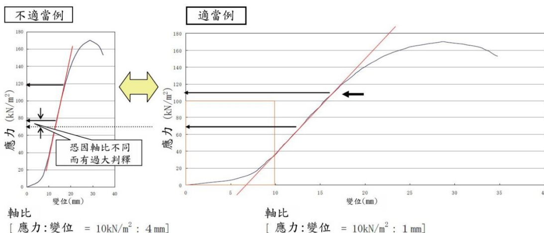
附圖 1-6 漸近線取軸法
