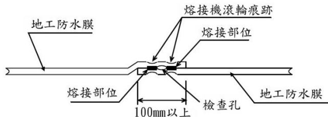
使用自走式熔接機之熔接
