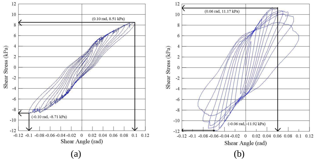
附圖 3-4 試驗結果之代表性剪應力與剪變形角對應圖
