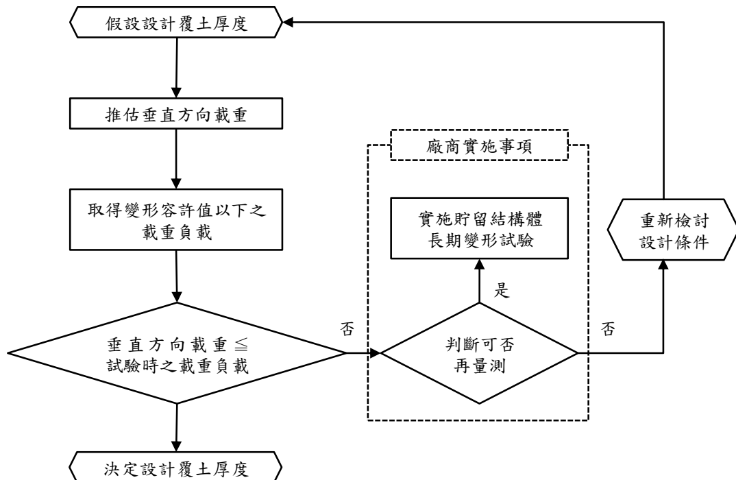
圖-解 3.7.3-1 長期性能試算流程(垂直方向)圖
