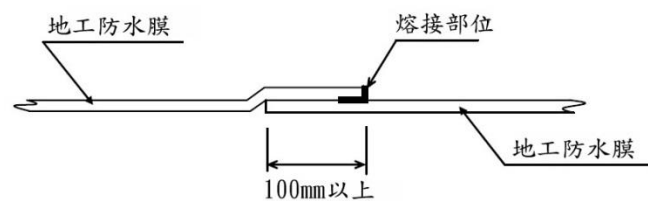
圖-解 4.2.7-2 地工防水膜之熔接示意圖
