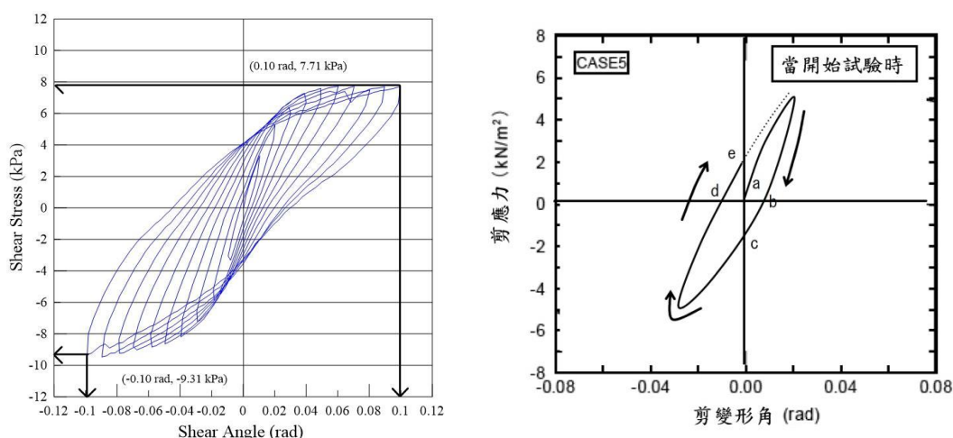
附圖 3-3 往復荷載抗剪試驗之曲線圖(例)
