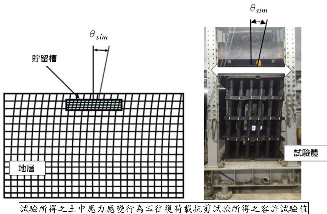
附圖 3-1 往復荷載抗剪性能評估示意圖
