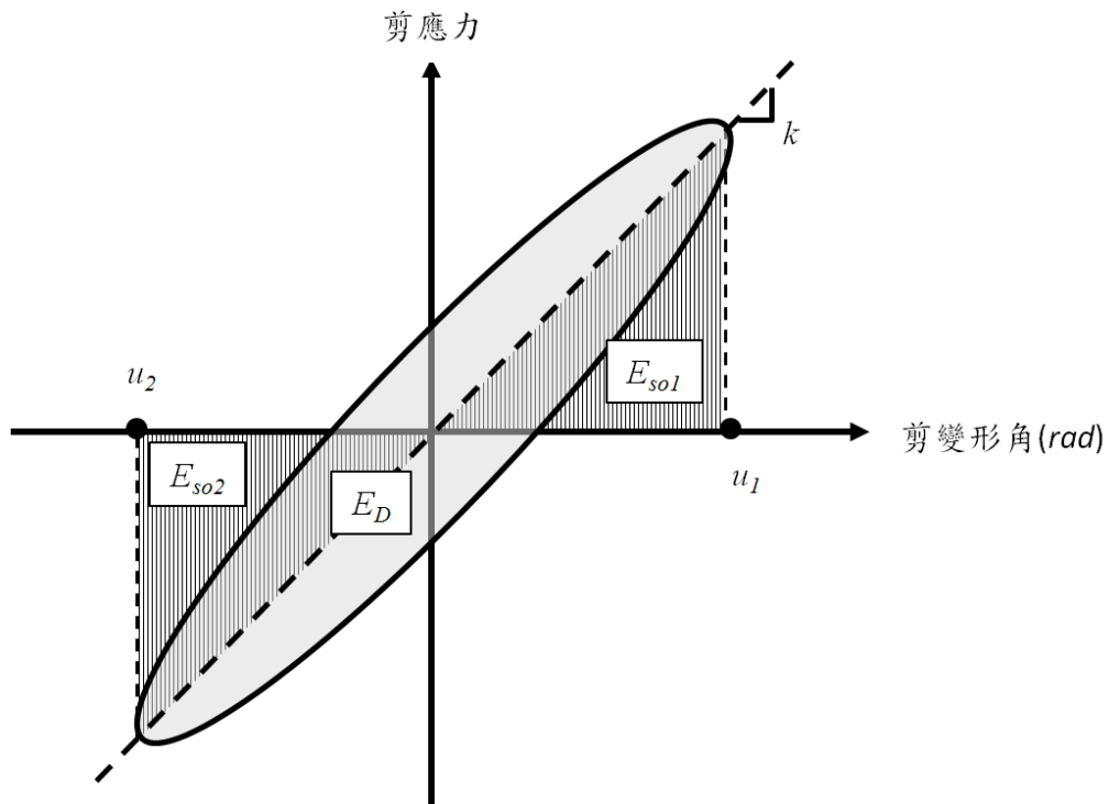
附圖 3-5 代表性彈簧與阻尼器併聯系統能量與應變量對應圖
