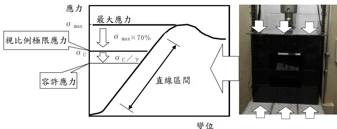
附圖 1-5 應力—位移曲線 (示意圖)
