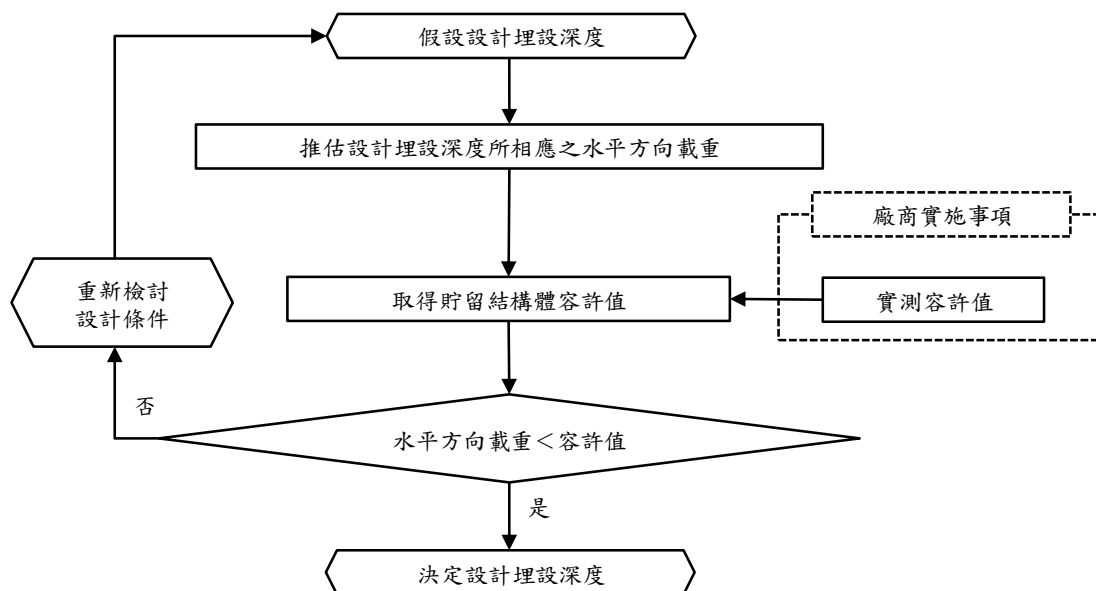
圖-解 3.7.2-5 水平方向之強度性能試算流程圖
