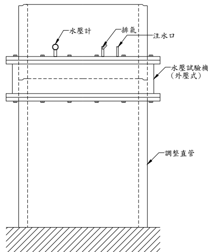
接頭部水密性試驗示意圖
