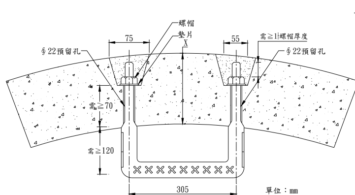
貫穿式塑膠包覆人孔踏步組裝方式示意圖
